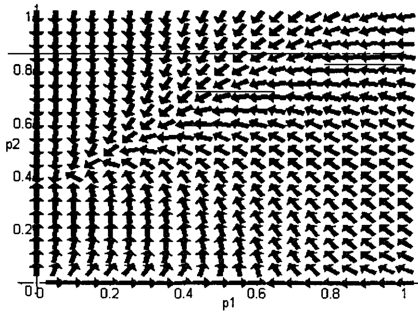
Figura II.5.11b: Campo de direcciones
