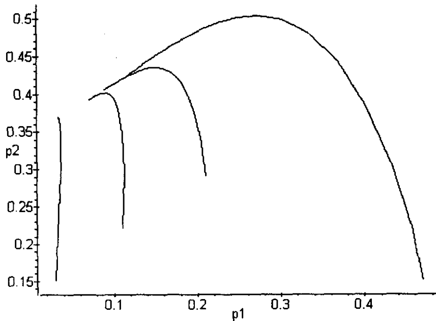
Figura II.5.11d: Trayectorias en plano fase
