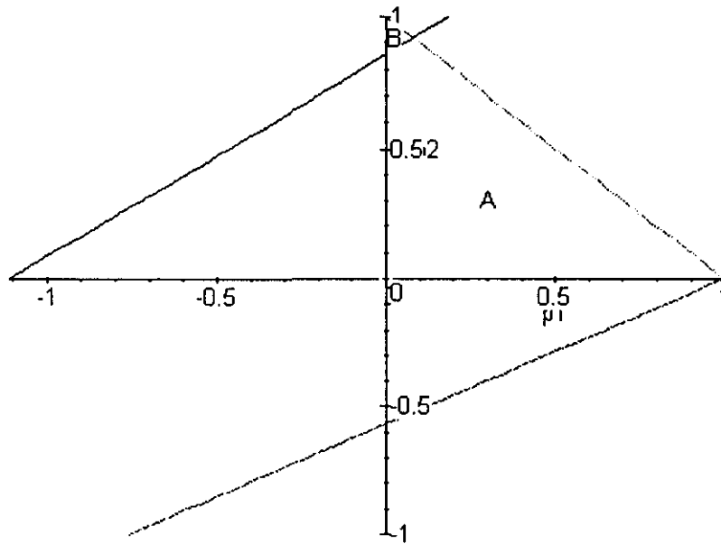
Figura III.6.27a: Regiones en plano fase
