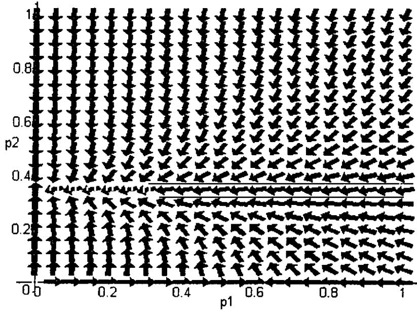
Figura II.5.4b: Campo de direcciones
