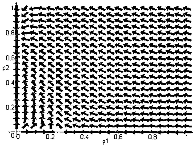
Figura II.5.10b: Campo de direcciones
