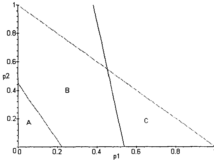
Figura II.6.3a: Regiones en plano fase
