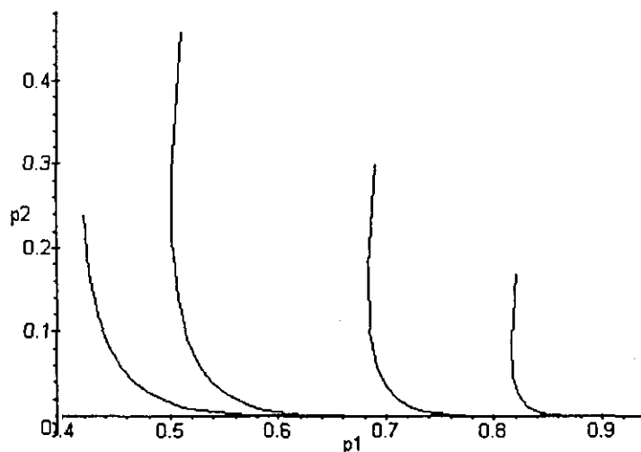
Figura II.5.6d: Trayectorias en plano fase
