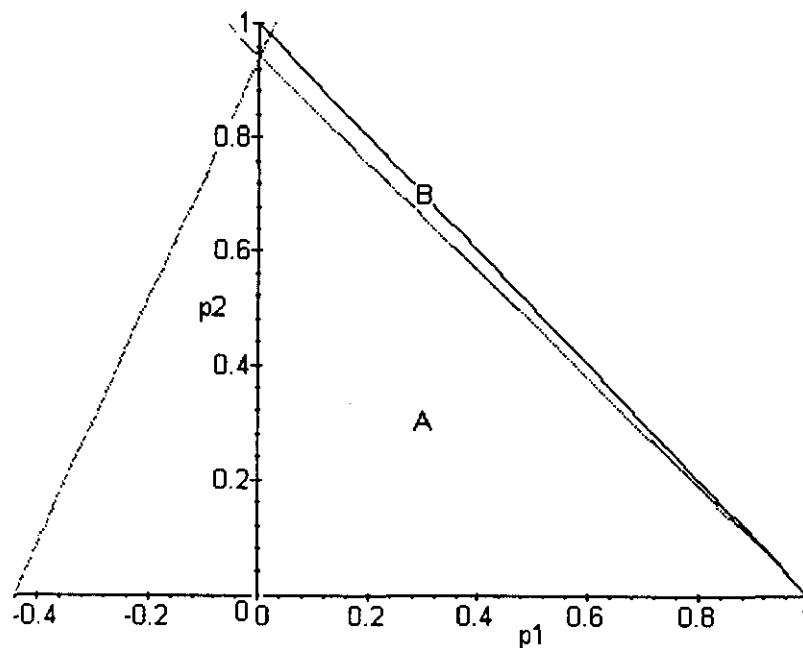
Figura III.6.20a: Regiones en plano fase
