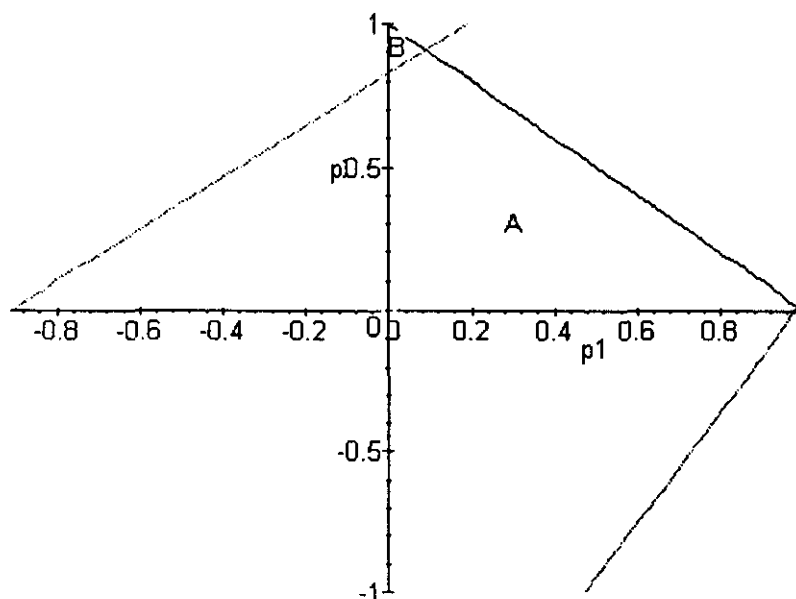
Figura III.6.6a: Regiones en plano fase
