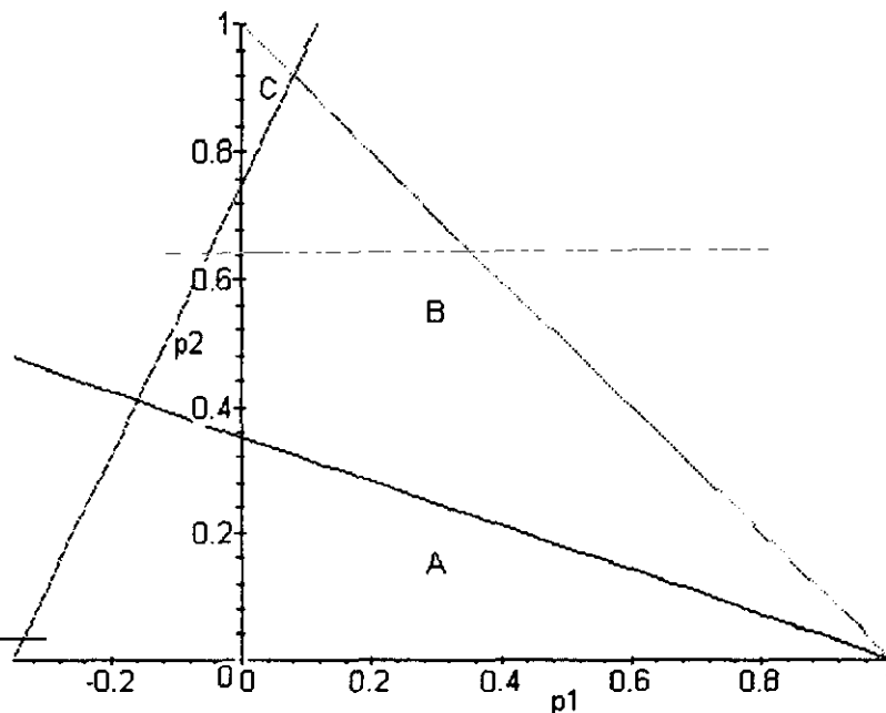
Figura III.6.21a: Regiones en plano fase
