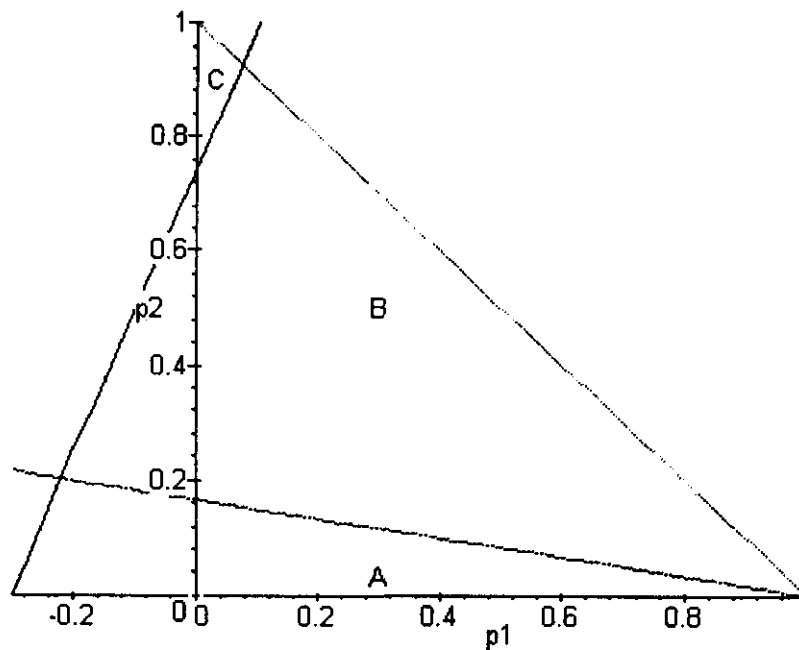
Figura III.6.3a: Regiones en plano fase
