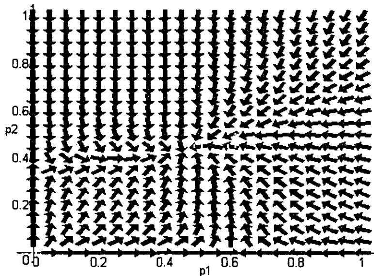
Figura II.5.9b: Campo de direcciones
