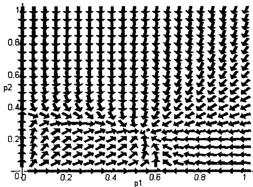
Figura II.6.1b: Campo de direcciones
