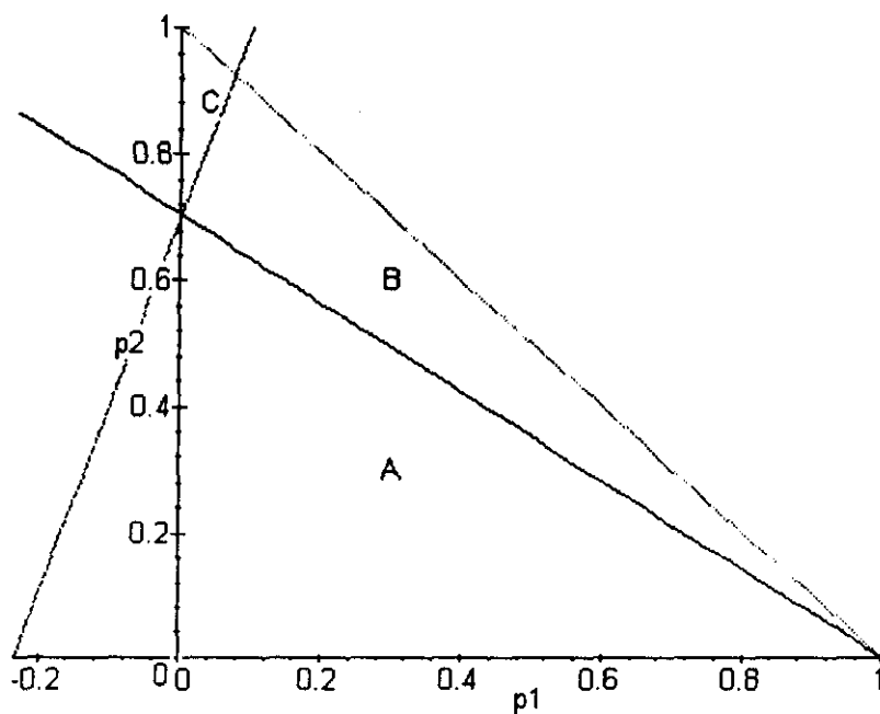
Figura III.6.2a: Regiones en plano fase
