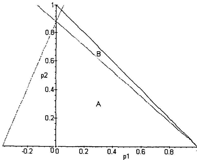
Figura III.6.22a: Regiones en plano fase
