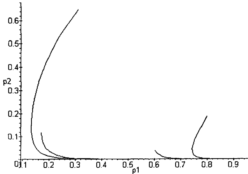
Figura II.5.7d: Trayectorias en plano fase
