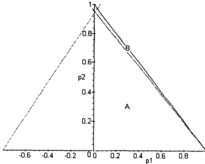
Figura III.6.29a: Regiones en plano fase
