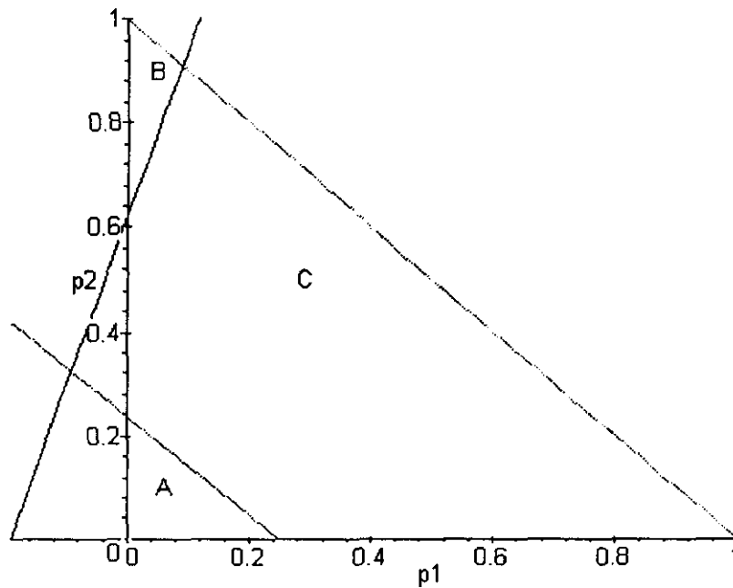
Figura II.5.10a: Regiones en plano fase
