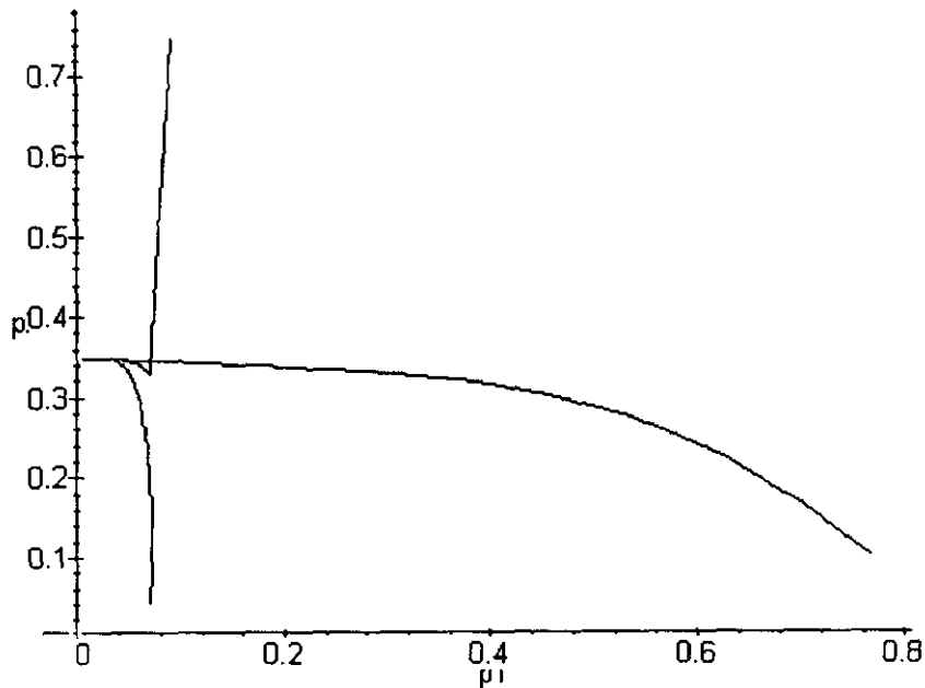
Figura II.5.4d: Trayectorias en plano fase
