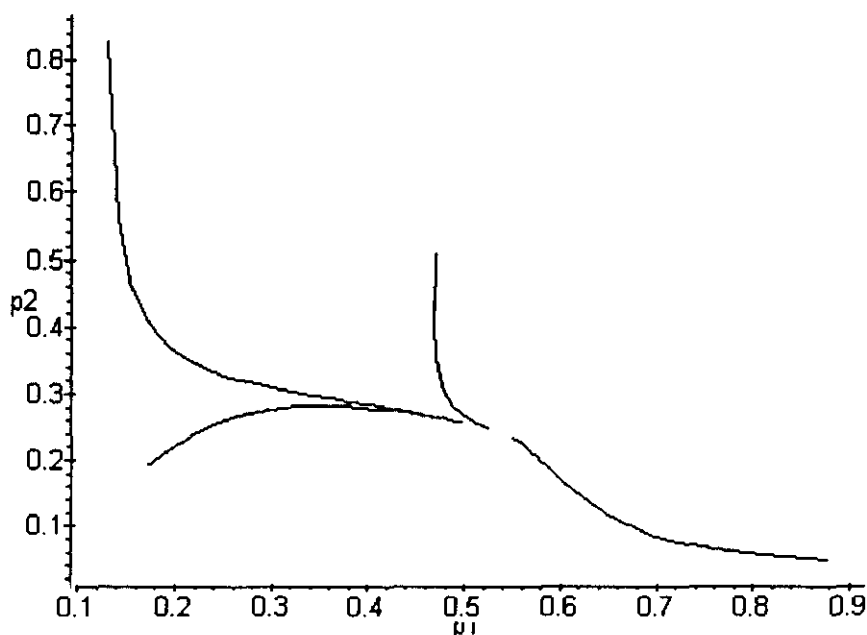
Figura II.5.1d: Trayectorias en plano fase
