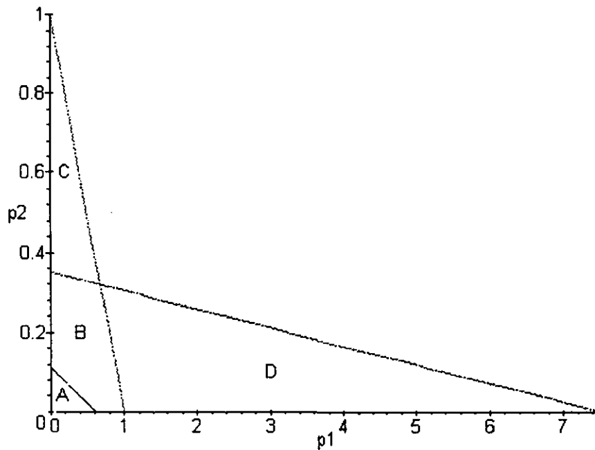
Figura II.5.4a: Regiones en plano fase
