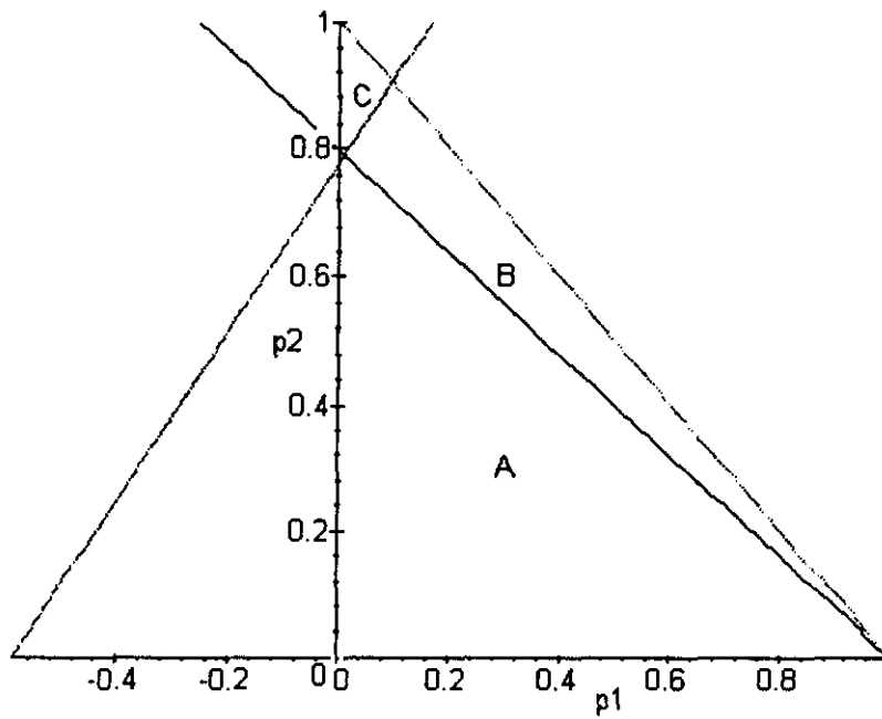
Figura III.6.1a: Regiones en plano fase
