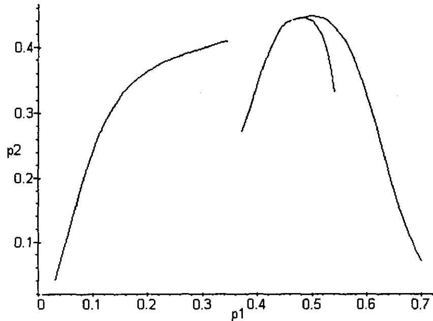
Figura II.5.9d: Trayectorias en plano fase
