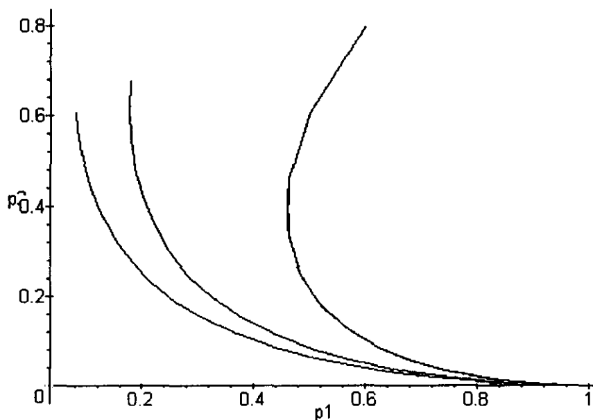
Figura II.5.8d: Trayectorias en plano fase
