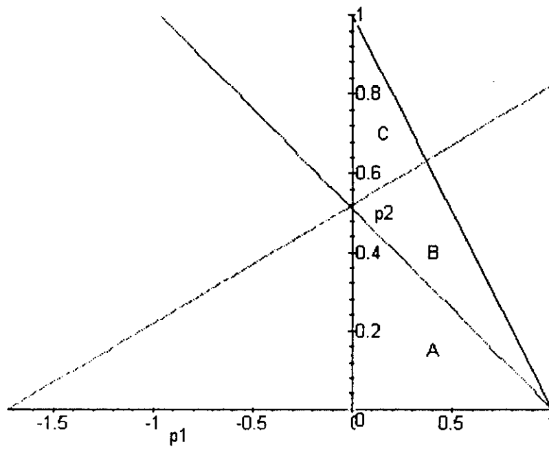
Figura III.6.15a: Regiones en plano fase
