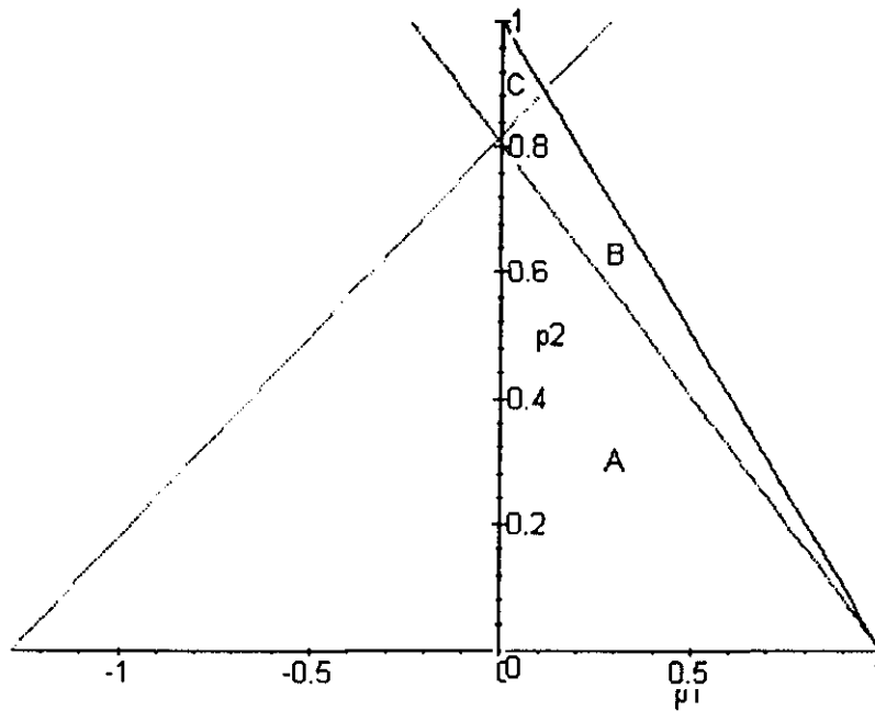
Figura III.6.30a: Regiones en plano fase
