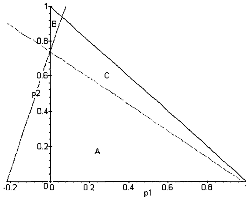
Figura II.6.8a: Regiones en plano fase
