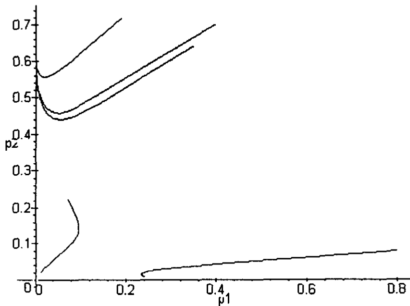
Figura II.5.2d: Trayectorias en plano fase
