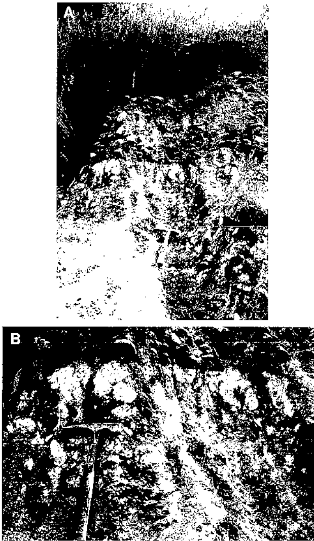
Figura 6.- Suelo de la terraza alta (perfil 1) junto al cortijo del Marqués de la Merced (longitud del martillo: 28 cm). Fotografía A: Horizontes superiores del perfil, Ap, AB, Bt, k y 2Bt, k. La discontinuidad estratigráfica entre dos secuencias sedimentarias de la terraza determina el cambio tan brusco de los dos últimos horizontes. Fotografía B: Detalle de carbonatación secundaria con carácter nodular en el perfil anterior.
