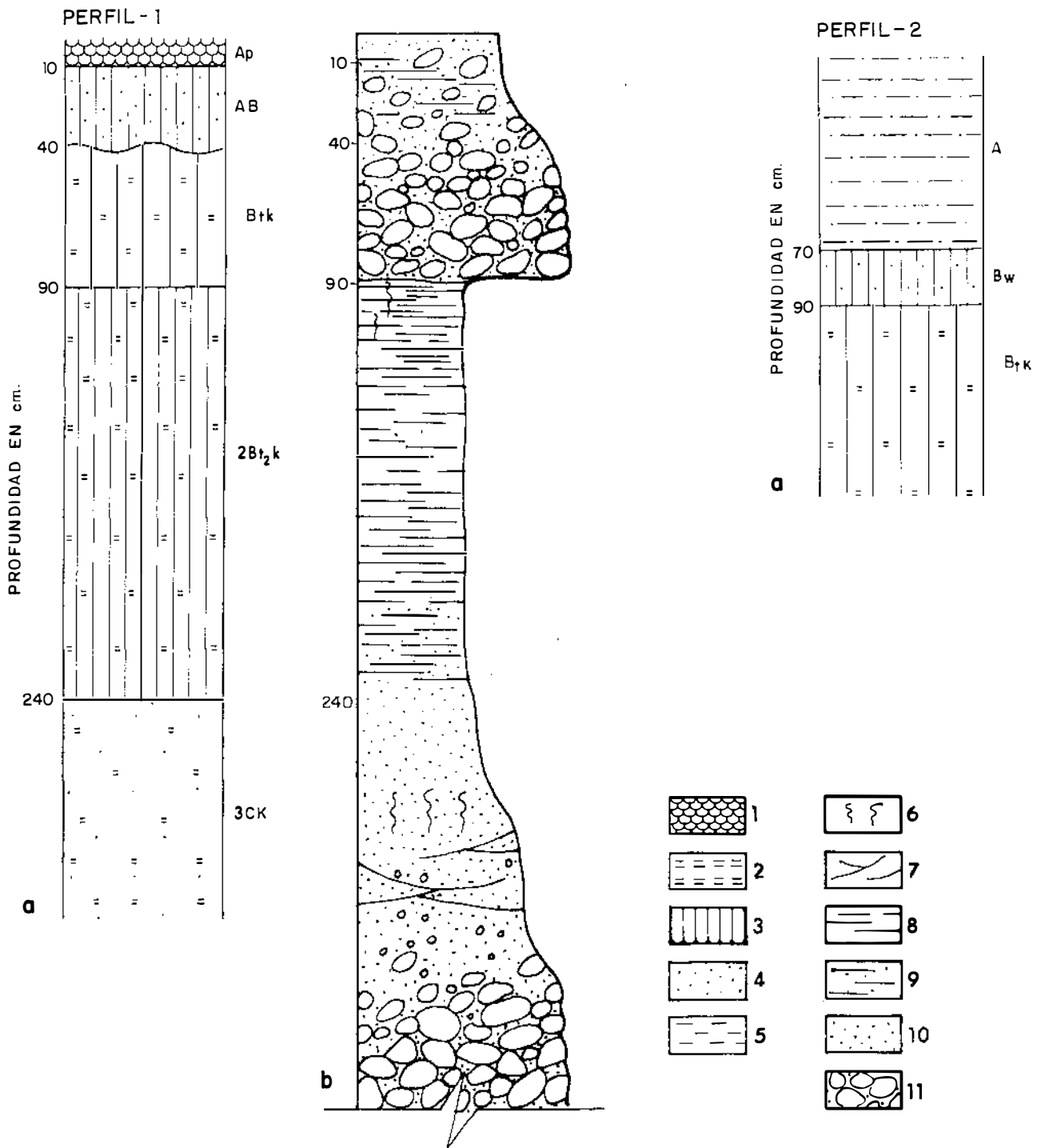
Figura 5.- Suelos de las terrazas altas. Los dos perfiles se encuentran sobre el mismo nivel de terraza distanciados unos 2 km. La diferencia entre ambos estriba en el desarrollo de los horizontes superficiales, bastante mayor en el perfil 2. Al perfil 1 se le adjunta su columna estratigráfica. Leyenda: a) Perfiles edáficos: 1, Horizonte A con materia orgánica; 2, Acumulación de carbonato cálcico; 3, Horizonte Bt con estructura prismática; 4, Horizonte arenoso; 5, Acumulación de arcilla; b) Columna estratigráfica: 6, Bioturbación; 7, Estratificación cruzada; 8, Arcilla; 9, Limos; 10, Arenas; 11, Conglomerados.
