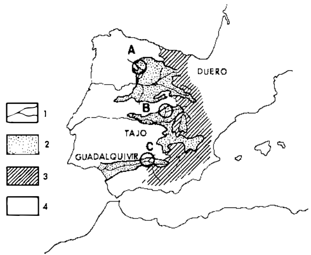
Figura 9.- Situación de las secuencias edáficas estudiadas por Herail (1979) (A), Vaudour (1979), Gallardo et al. (1987) (B) y en este artículo (C). Leyenda: 1, Red fluvial; 2, Cuencas terciarias; 3, Área fuente carbonatada; 4, Área fuente silíceo.
