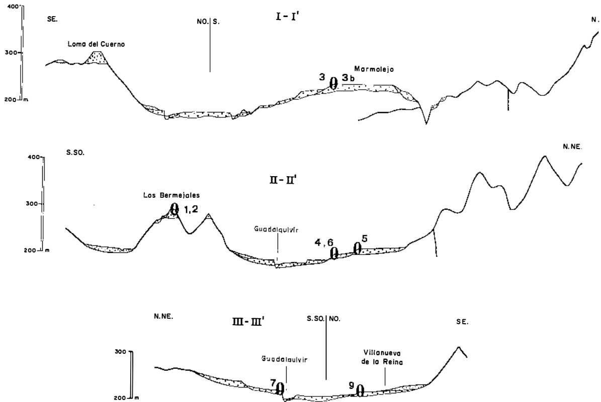
Figura 4.- Cortes geomorfológicos (ver situación en figura 5) y posición de los suelos estudiados.
