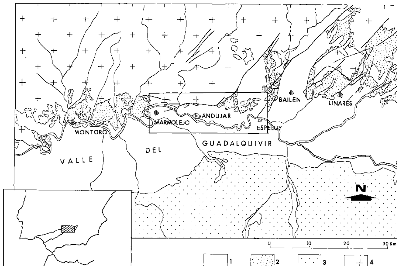
Figura 1.- Situación y contexto geológico regional. Leyenda: 1, Cenozoico; 2, Mesozoico de la periferia del Macizo Hespérico; 3, Terrenos subbéticos; 4, Macizo Hespérico.
