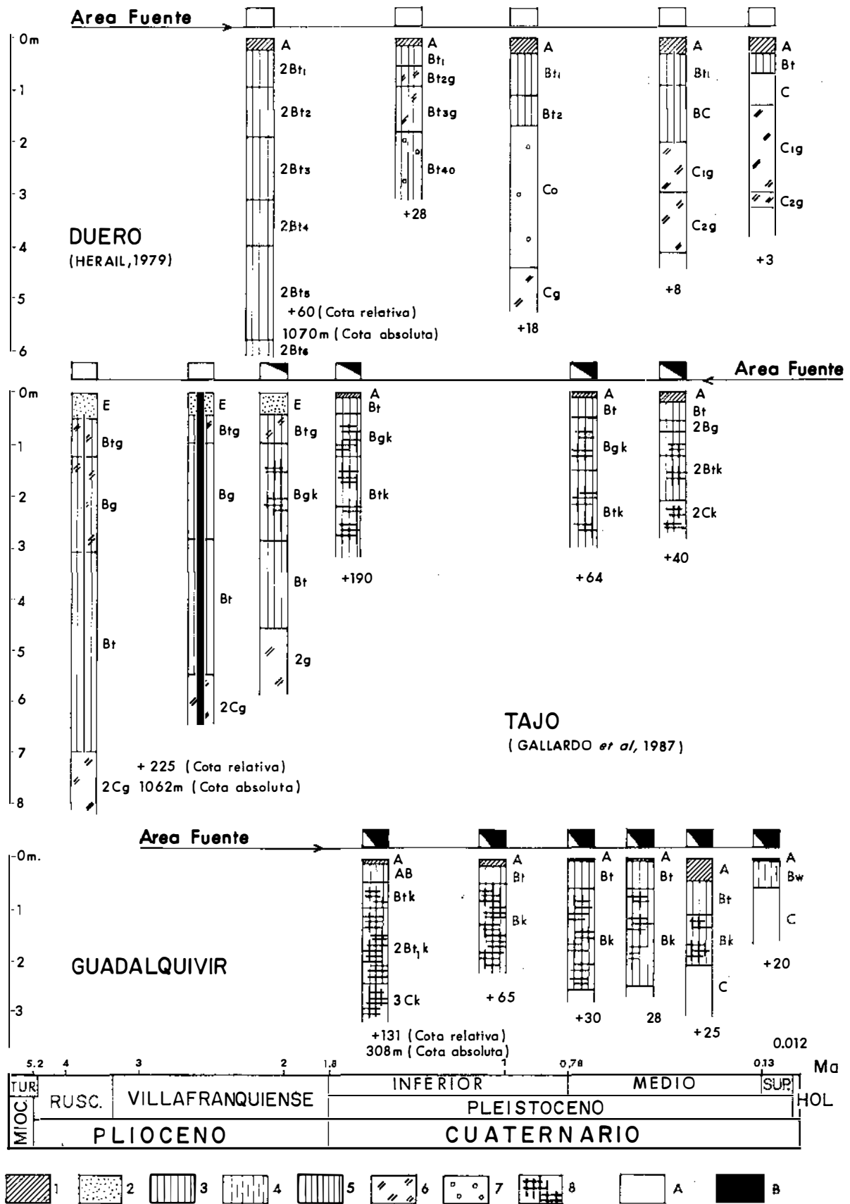
Figura 10.- Gráfico comparativo de las tres secuencias edáficas emplazadas. Leyenda: Pérfiles edáficos: 1, horizonte A; 2, horizonte E; 3, horizonte B; 4, horizonte C; 5, horizonte argílico; 6, hidromorfías; 7, acumulaciones de Fe; 8, carbonato. Area fuente: A, silíceas; B, carbonatadas (la importancia de una u otra area fuente se expresa gráficamente en el cuadro que encabeza cada perfil).
