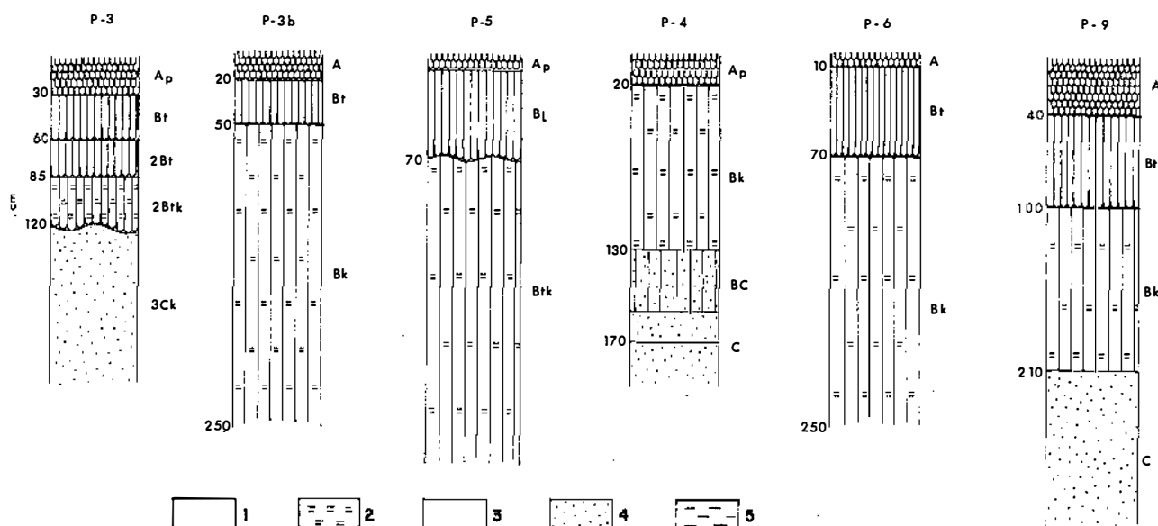
Figura 7.- Suelos de las terrazas medias (profundidad de los horizontes del suelo en cm). Leyenda: 1, Horizonte A con materia orgánica; 2, Acumulación de carbonato cálcico; 3, Horizonte Bt con estructura prismática; 4, Horizonte arenoso; 5, Acumulación de arcilla.
