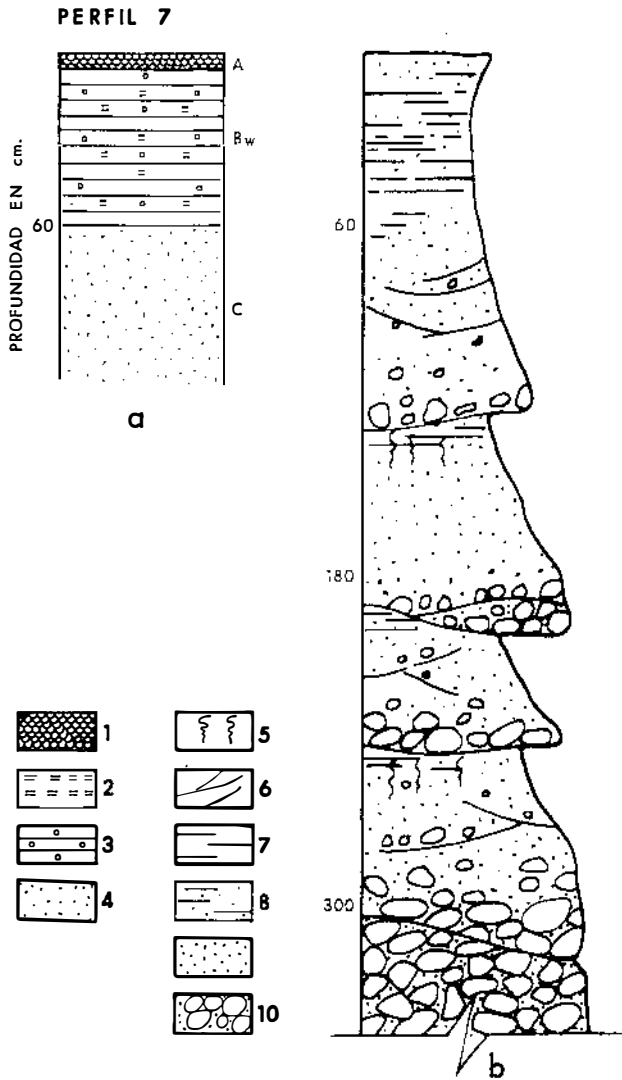
Figura 8.- Suelo y columna estratigráfica correspondiente en una terraza baja (profundidad de los horizontes del suelo en cm), Leyenda: a) Perfil edáfico: 1, Horizonte A con materia orgánica; 2, Acumulación de carbonato cálcico; 3, Horizonte Bw ; 4, Horizonte arenoso; b) Columna estratigráfica: 5, Bioturbación; 6, Estratificación cruzada; 7, Arcilla; 8, Limos; 9, Arenas; 10, Conglomerados.
