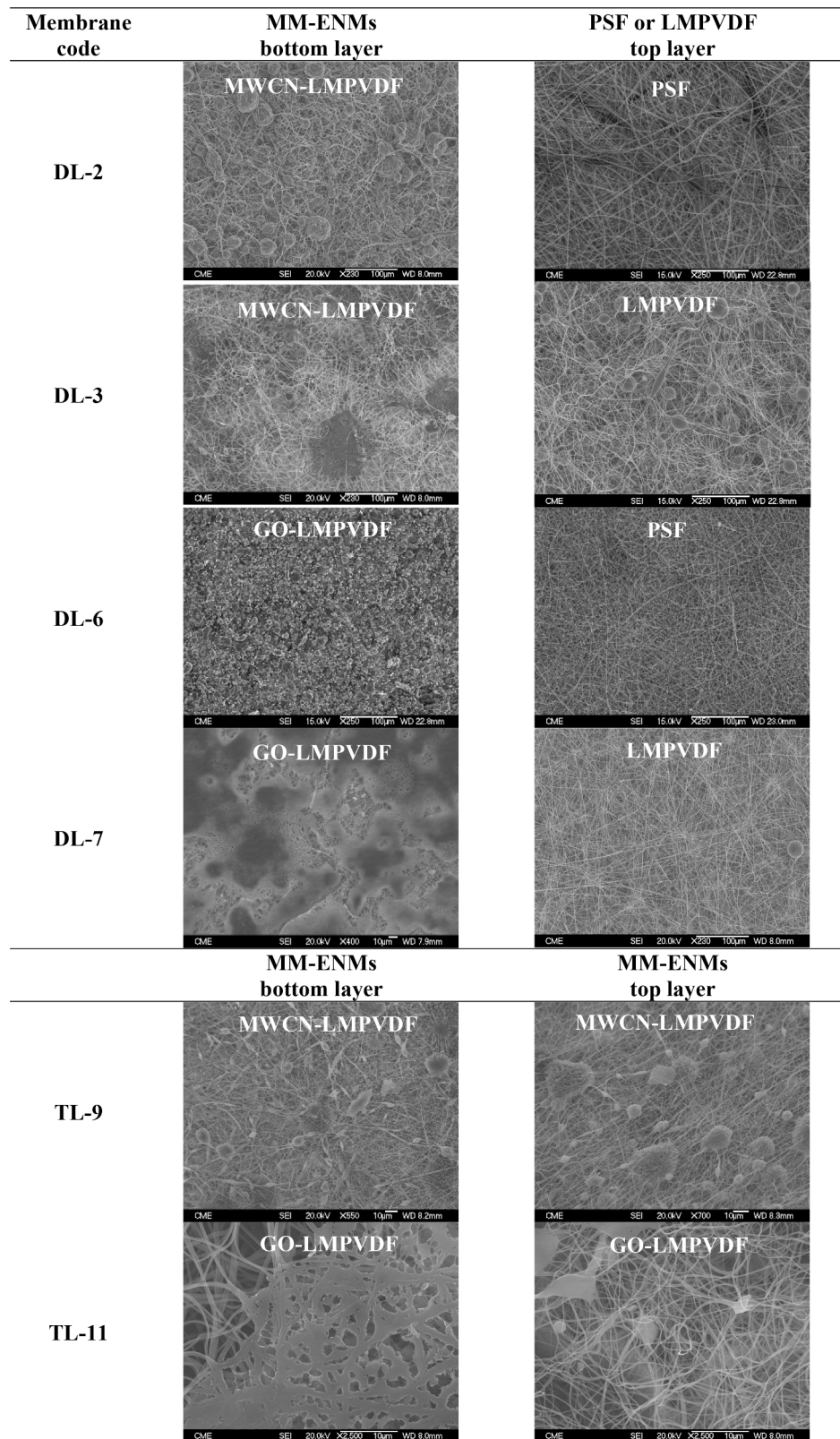
Fig. 9. FESEM images of DL-MM-ENMs and TL-MM-ENMs.
