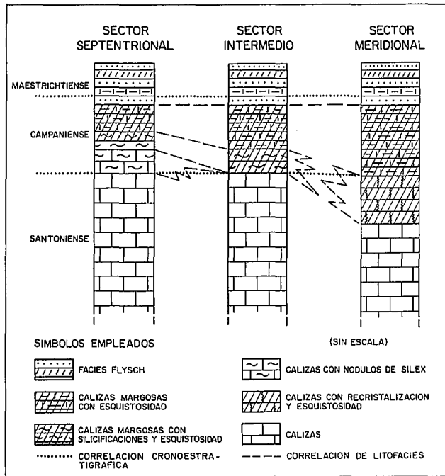
Fig. 6.—Esquema de las variaciones de facies entre los sectores meridional y septentrional.
