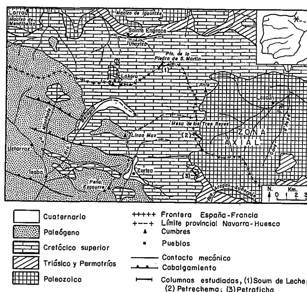
Fig. 1.—Entorno geológico y localización de las columnas estratigráficas estudiadas.
