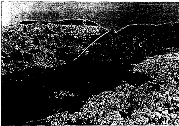
Fig. 8.—Contacto entre las calizas del Santoniense (S) y las calizas con nódulos de sílex del Campaniense (C), en este caso afectadas por una falla (F). Vertiente septentrional del Pto. de la Piedra de San Martín.
