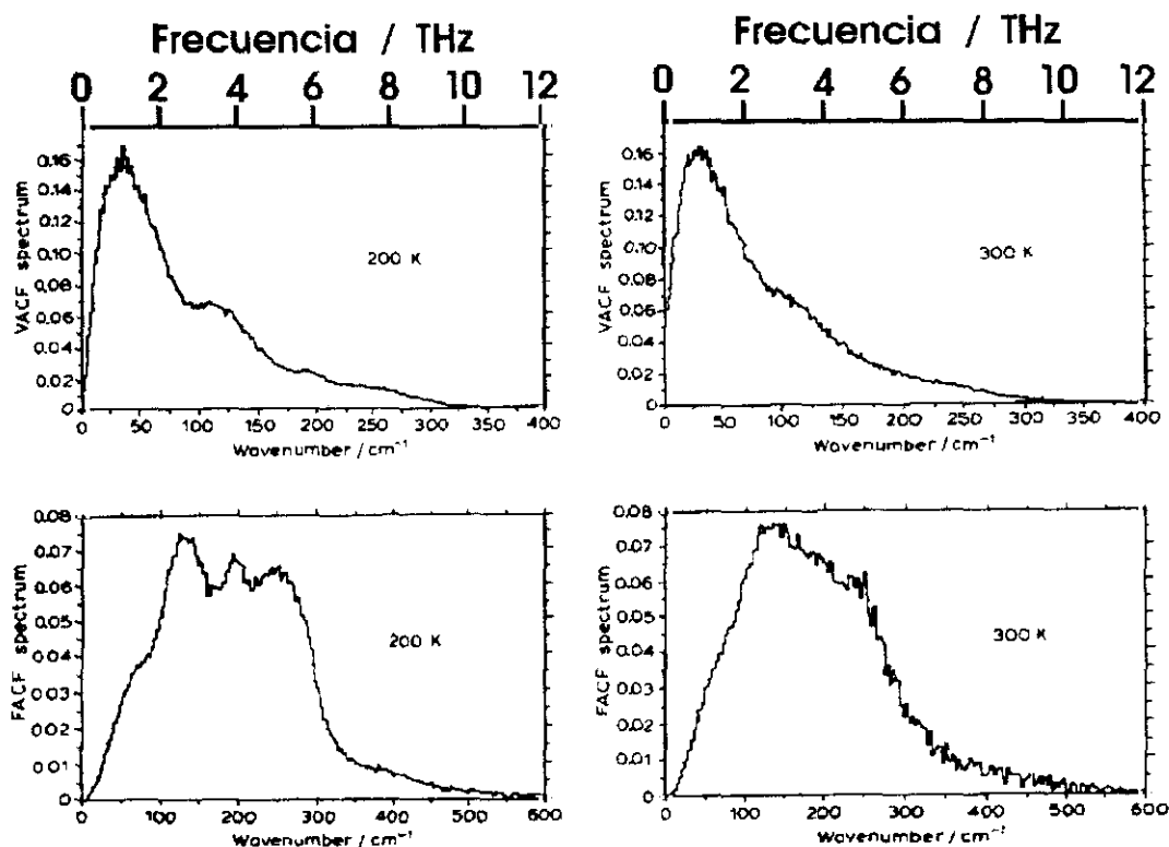
Figura 7.7: Transformadas de Fourier de las FACVs y FACFs normalizadas a 200 y 300 K. Nota: 33.35 \text{ cm}^{-1} equivalen a 1 THz.
