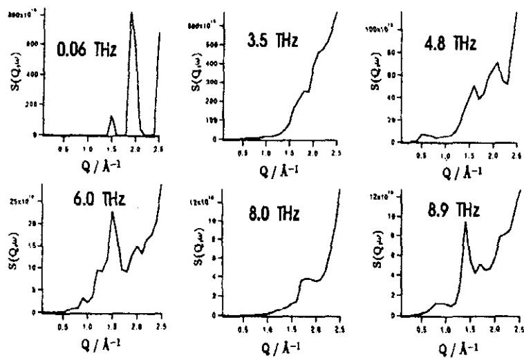
Figura 7.19: Factores de estructura inelásticos: S(Q, \omega = \text{cte}) , para valores de la frecuencia coincidentes con los picos más intensos observados en la densidad de estados calculada mediante dinámica reticular.
