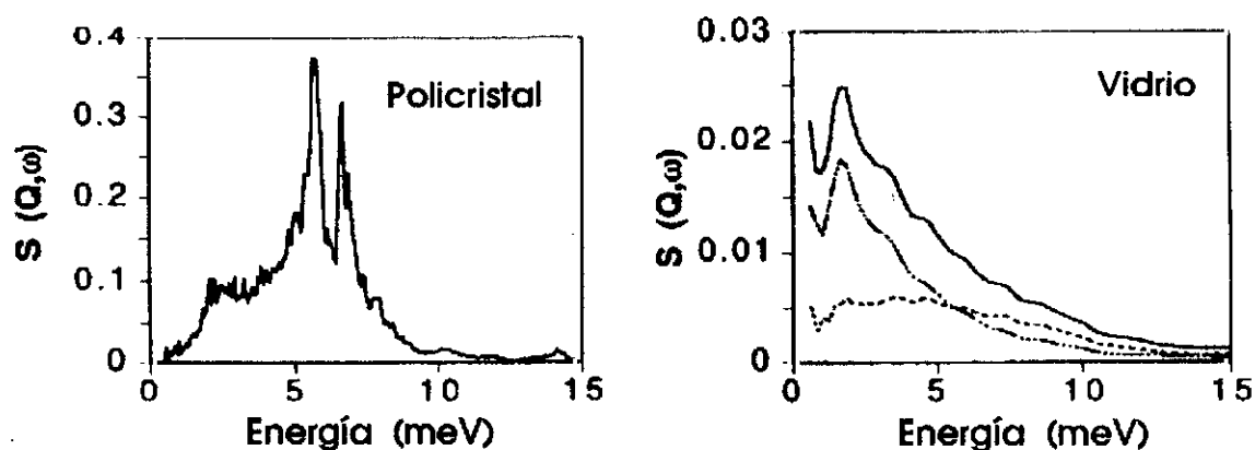
Figura 7.20: Factores de estructura dinámicos incoherentes, S_{inc}(Q, \omega) , calculados a partir de las densidades de estados, Z(\omega) , obtenidas por dinámica reticular para el policristal (izquierda) y dinámica molecular para el vidrio (derecha) para un valor de Q = 2.5 \text{ \AA}^{-1} . En el caso del vidrio, la función total (línea continua) se ha descompuesto en sus componentes rotacional (línea discontinua) y de centros de masa (línea a trazos y puntos). Obsérvese como el pico de baja frecuencia visible en el vidrio se debe a la componente de centros de masa.
