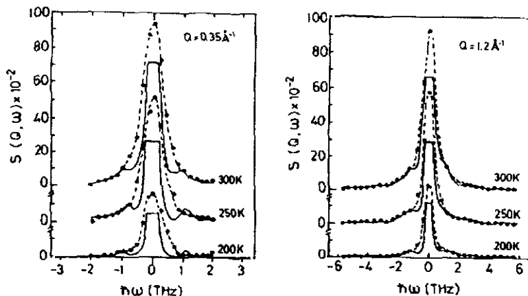
Figura 8.5: Dependencia de los espectros reconstruidos con la temperatura para Q = 0.35 y 1.2 \text{ \AA}^{-1} . Los puntos unidos por líneas discontinuas corresponden a los espectros medidos; mientras que las líneas continuas representan los espectros reconstruidos.
