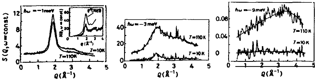
Figura 8.14: Intensidades inelásticas en función de Q para las dos temperaturas extremas y tres valores de la energía. En el recuadro se muestran las intensidades calculadas por medio de la aproximación de Buchenau et al. para \hbar\omega = -3 (círculos) y -6 meV (línea continua inferior) junto con Q^2 S(Q) (línea continua superior). Las líneas continuas se han trazado como ayuda visual.
