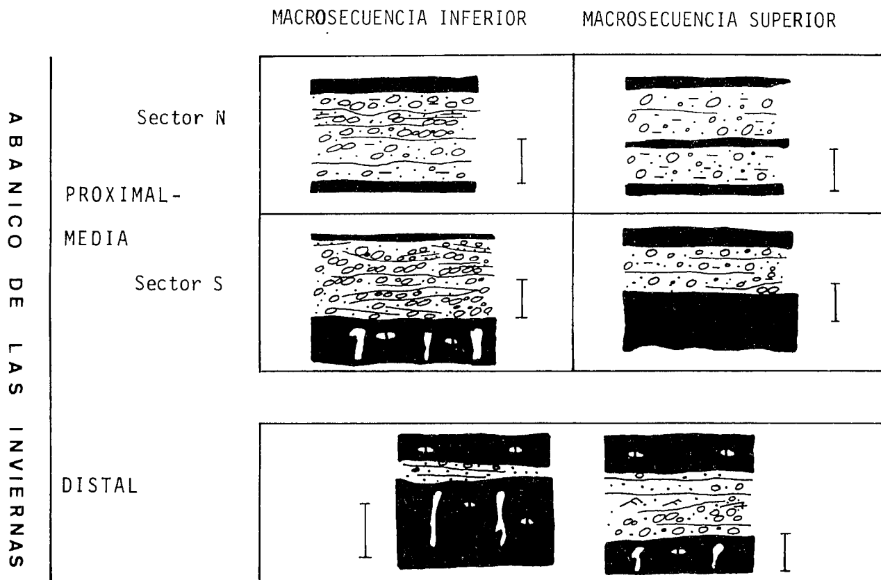
Fig. 10.-Asociaciones de facies reconocidas en el abanico de Las Inviernas. La barra que figura como escala equivale a 1 m. Fig. 10.-Facies assemblages of Las Inviernas fan. Scale bar = 1 m.
