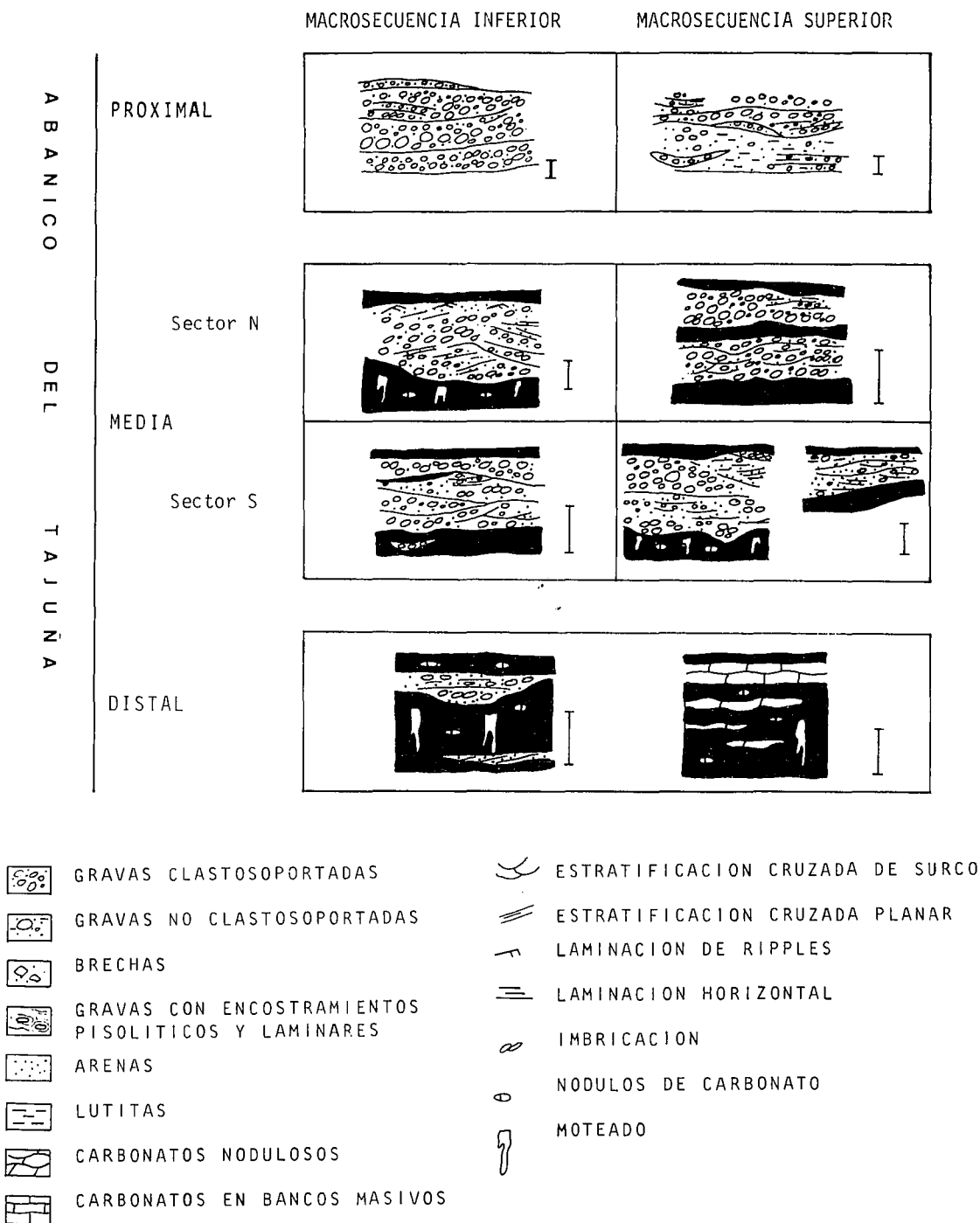
Fig. 5.-Asociaciones de facies reconocidas en el abanico del Tajuña. La barra que figura como escala equivale a 1 m. Fig. 5.-Facies assemblages of the Tajuña fan. Scale bar = 1 m.
