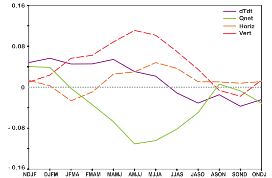
(b) HB Atl3 [20W-0,3N-3S] Atlantic Niño
