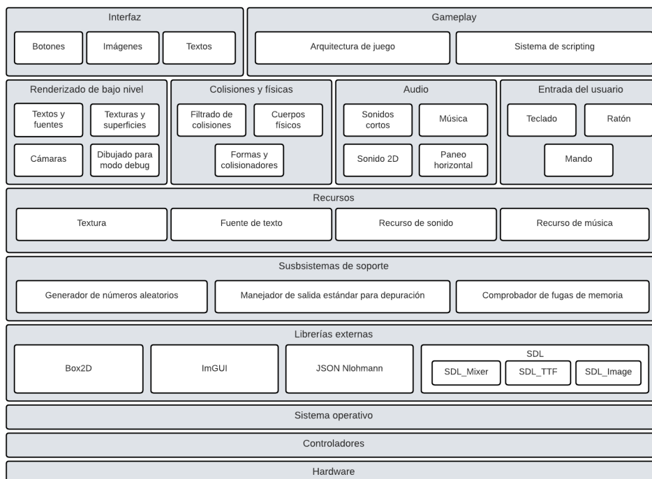
Figura 4.1: Arquitectura del motor.
