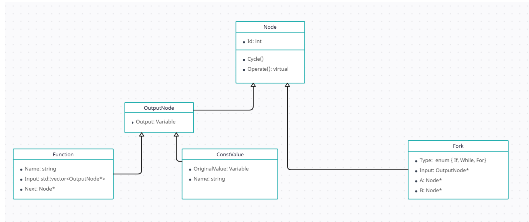
Figura 4.7: Diagrama UML con la estructura de clases de los nodos del scripting
