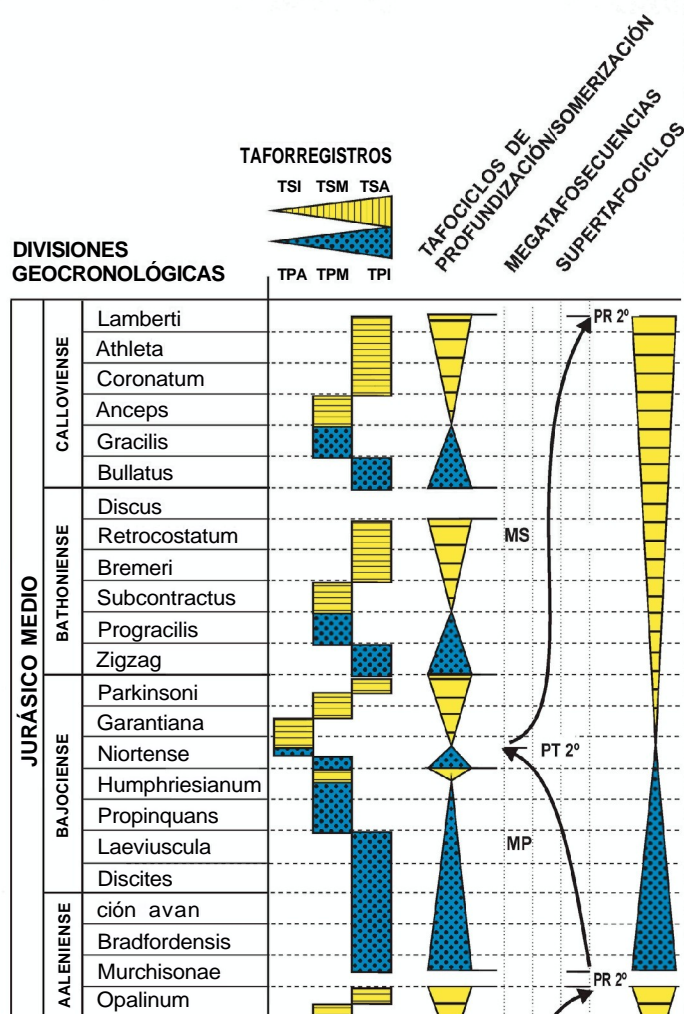
Figura 13. Taforregistros, tafociclos de profundización/somerización y megatafosecuencias identificadas en las asociaciones registráticas de ammonites del Jurásico Medio de las plataformas Castellana, Aragonesa y de Tortosa. MP= megatafosecuencia de profundización. MS= megatafosecuencia de somerización. TPI= taforregistro de profundización incipiente. TPM= taforregistro de profundización media. TPA= taforregistro de profundización avanzada. TSI= taforregistro de somerización incipiente. TSM= taforregistro de somerización media. TSA= taforregistro de somerización avanzada. PT 2°= pico transgresivo de segundo orden. PR 2° = pico regresivo de segundo orden.
