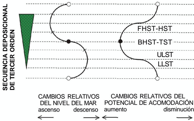
Figura 7. Sistemas deposicionales y fases sucesivas durante el desarrollo de las secuencias deposicionales de tercer orden. LLST = sistema deposicional inferior de bajo nivel ( lower lowstand systems tract ). ULST = sistema deposicional superior de bajo nivel ( upper lowstand systems tract ). BHST o TST = sistema deposicional retrogradacional de alto nivel ( backstepping highstand systems tract o transgressive systems tract ). FHST o HST = sistema deposicional progradacional de alto nivel ( forestepping highstand systems tract o highstand systems tract ).
