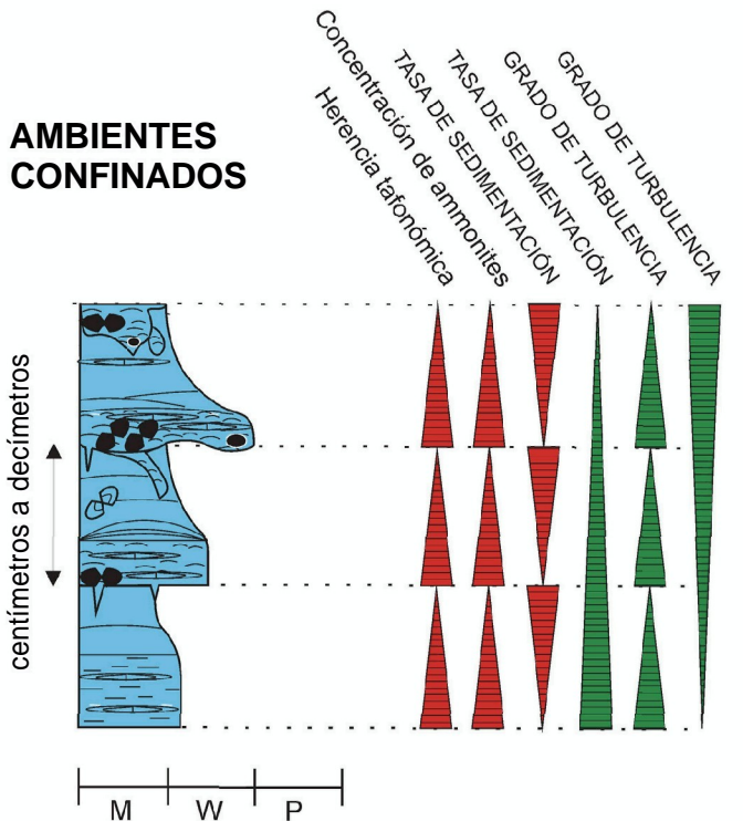
Figura 2. Secuencias elementales frecuentes en las parasecuencias del Jurásico Medio de la Cordillera Ibérica, con indicación de las variaciones en el grado de turbulencia y en la tasa de sedimentación. El grado de turbulencia aumenta y la tasa de sedimentación disminuye durante el desarrollo de las parasecuencias en los ambientes de plataforma externa carbonática. La sedimentación de fondo que da lugar a estas secuencias elementales también experimenta variaciones en el grado de turbulencia, inversamente proporcionales a la tasa de sedimentación. No obstante, el grado de turbulencia es creciente en los ambientes abiertos y decreciente en los ambientes confinados durante el desarrollo de las secuencias elementales. Debido a estas variaciones ambientales, durante el desarrollo de estas secuencias elementales, el grado de herencia tafonómica (estimado por la proporción de elementos reelaborados) y la concentración de los restos de ammonites aumentan en los ambientes abiertos, pero los valores de estos dos parámetros disminuyen en los ambientes confinados.
