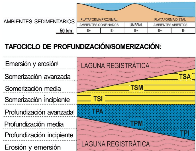
Figura 11 Los taforregistros de ammonites desarrollados en las plataformas epicontinentales carbonáticas durante un tafociclo de profundización/somerización presentan caracteres más variados en las áreas distales y deprimidas que en las áreas proximales y someras. Los taforregistros de profundización incipiente (TPI) y los de somerización avanzada (TSA) sólo se desarrollaron en las áreas distales de la plataforma. TPI= taforregistro de profundización incipiente. TPM= taforregistro de profundización media. TPA= taforregistro de profundización avanzada. TSI= taforregistro de somerización incipiente. TSA= taforregistro de somerización media. TSA= taforregistro de somerización avanzada.
