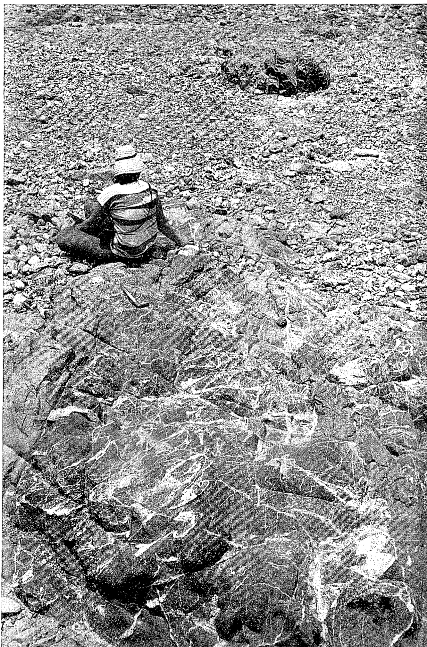
Fig. 3.-Detalle de un afloramiento de rocas ultramáficas con su "net-work" feldespático. Fig. 3.-Detail of the dense feldspatic net-work of the ultramafic rocks.
