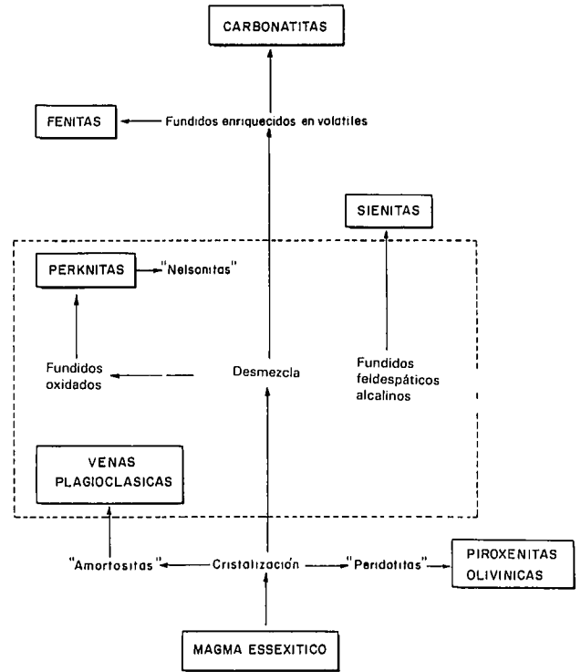
Fig. 8.-Esquema petrogenético del complejo ultramáfico-carbonatítico de Amanay.
