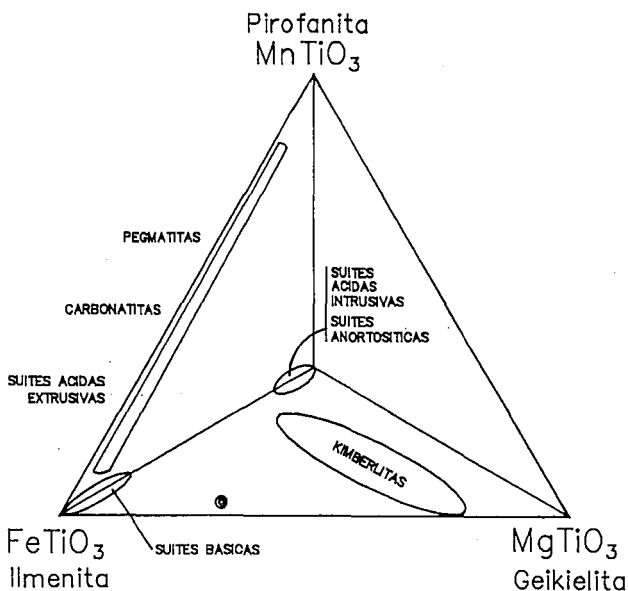
Fig. 7.-Situación de la ilmenita (Análisis n.º 4, Tabla 1) en el diagrama MnTiO 3 -FeTiO 3 -MgTiO 3 (Haggerty, 1976). Fig. 7.-Composition of the ilmenite (Analysis 4, Table 1) in the MnTiO 3 -FeTiO 3 -MgTiO 3 diagram (Haggerty, 1976).
