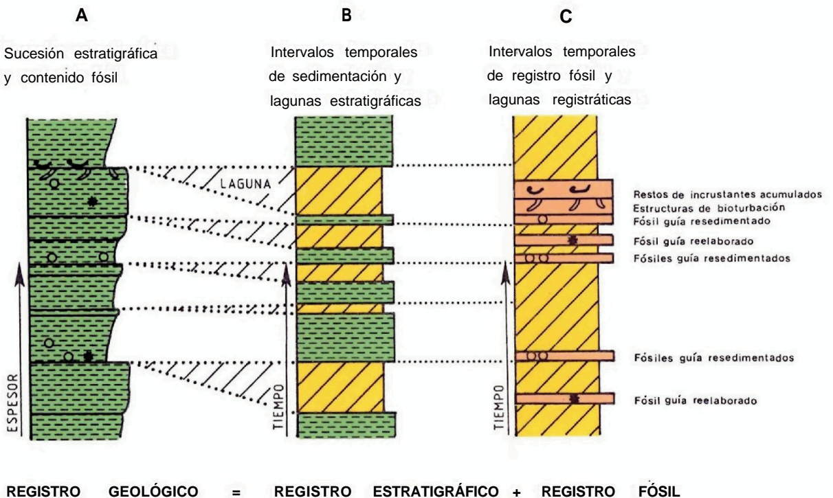
Fig. 6.—Relación entre los intervalos temporales de sedimentación (B) y los intervalos temporales de registro fósil (C) representados por una sucesión estratigráfica local y su contenido fósil (A). Para averiguar los intervalos temporales de registro fósil debe tenerse en cuenta que los fósiles acumulados son contemporáneos con el intervalo temporal de formación del correspondiente nivel estratigráfico, pero más recientes que los fósiles reelaborados y heredados del mismo nivel. La presencia de lagunas estratigráficas no garantiza la ausencia de registro fósil para el mismo intervalo temporal. En cualquier localidad, los intervalos temporales representados por los fósiles pueden corresponder a intervalos temporales sin registro estratigráfico. El registro fósil y el registro estratigráfico son dos componentes disociables del registro geológico, cuya dinámica de formación ha sido distinta, y para interpretarlos se requiere de conceptos estratigráficos, sedimentológicos y tafonómicos.
