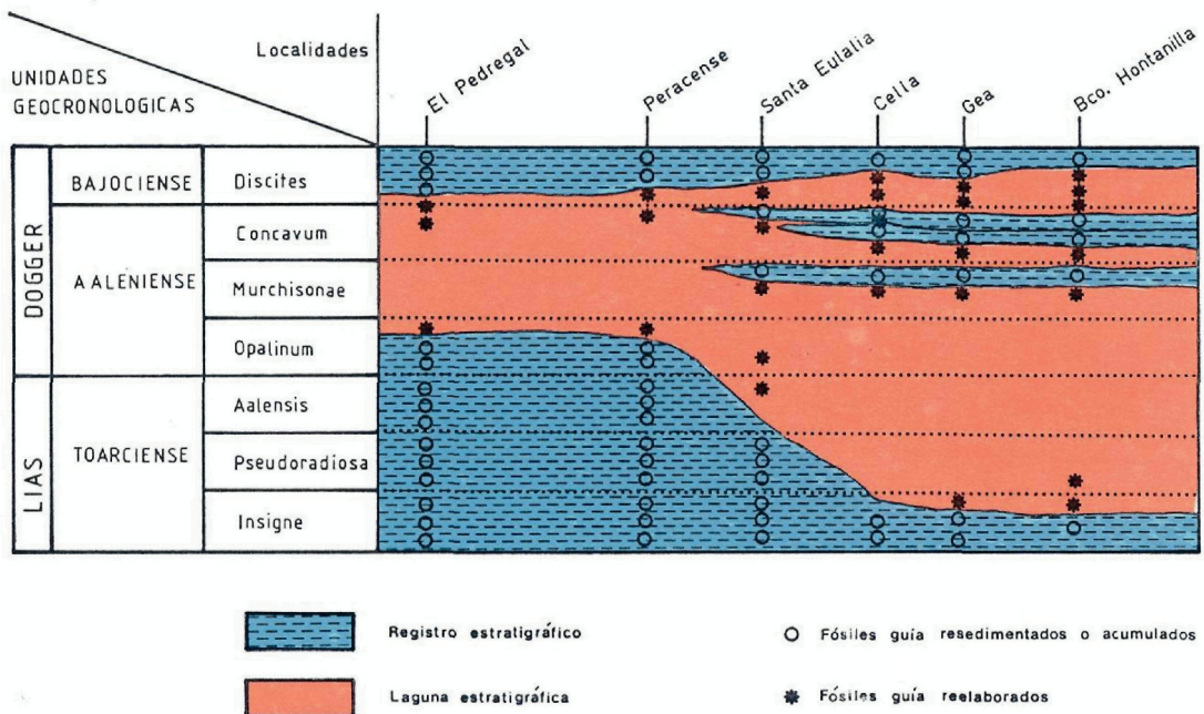
Fig. 4.—Distribución cronológica del registro estratigráfico y sus lagunas para el tránsito Lías-Dogger en varias localidades del sector central de la Cuenca Ibérica a lo largo de unos 60 kilómetros. Entre los fósiles guía utilizados para datar los cuerpos rocosos se han distinguido dos grupos que están indicados respectivamente con círculos (cuando se trata de elementos resedimentados o acumulados) y con asteriscos (si son elementos reelaborados). Las biozonas y cronozonas han podido ser identificadas teniendo en cuenta fósiles resedimentados. No obstante, los niveles de removilización son frecuentes y contienen fósiles heredados, a escala de zona o de piso. Debido a la reelaboración de moldes internos a partir de materiales preexistentes, los ammonites de algunos niveles son más antiguos que los materiales del nivel inmediatamente inferior. En algunas localidades hay fósiles guía reelaborados característicos de biozonas de las que no hay registro estratigráfico. En cualquier localidad donde hay fósiles reelaborados, las asociaciones de fósiles y los cuerpos rocosos que las contienen no representan el mismo intervalo temporal.
