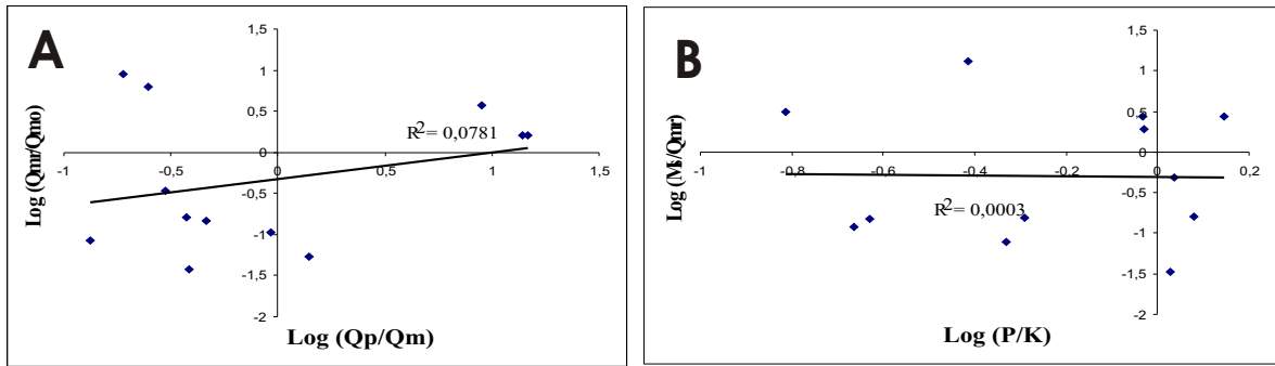
Fig. 12.- Log-ratio diagrams of (A) Qmr/Qmo vs Qp/Qm and (B) Ms/Qmr vs P/K for the Sierra de Matute Fm. (DS 2). Fig. 12.- Diagramas de los logaritmos de las relaciones (A) Qmr/Qmo vs Qp/Qm y (B) Ms/Qmr vs P/K para la Fm. Sierra de Matute (SD 2).
