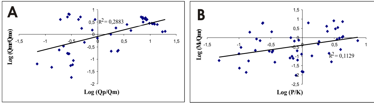
Fig. 10.- Log-ratio diagrams of (A) Qmr/Qmo vs Qp/Qm and (B) Ms/Qmr vs P/K for the Magaña Fm. (DS 2). Fig. 10.- Diagramas de los logaritmos de las relaciones (A) Qmr/Qmo vs Qp/Qm y (B) Ms/Qmr vs P/K para la Fm. Magaña (SD 2).
